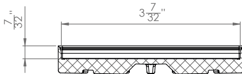
SECCIÓN A-A
