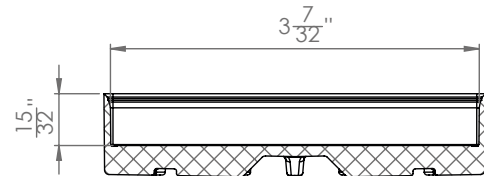
SECCIÓN A-A
